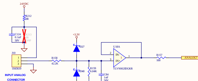
ANALOG INPUTS
