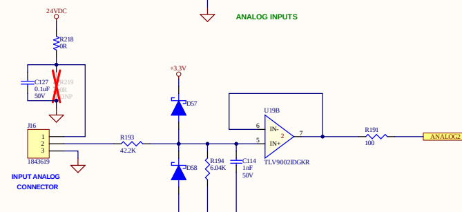
ANALOG INPUTS
